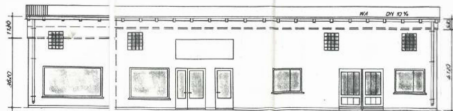
Hofansicht neu M 1 : 100
