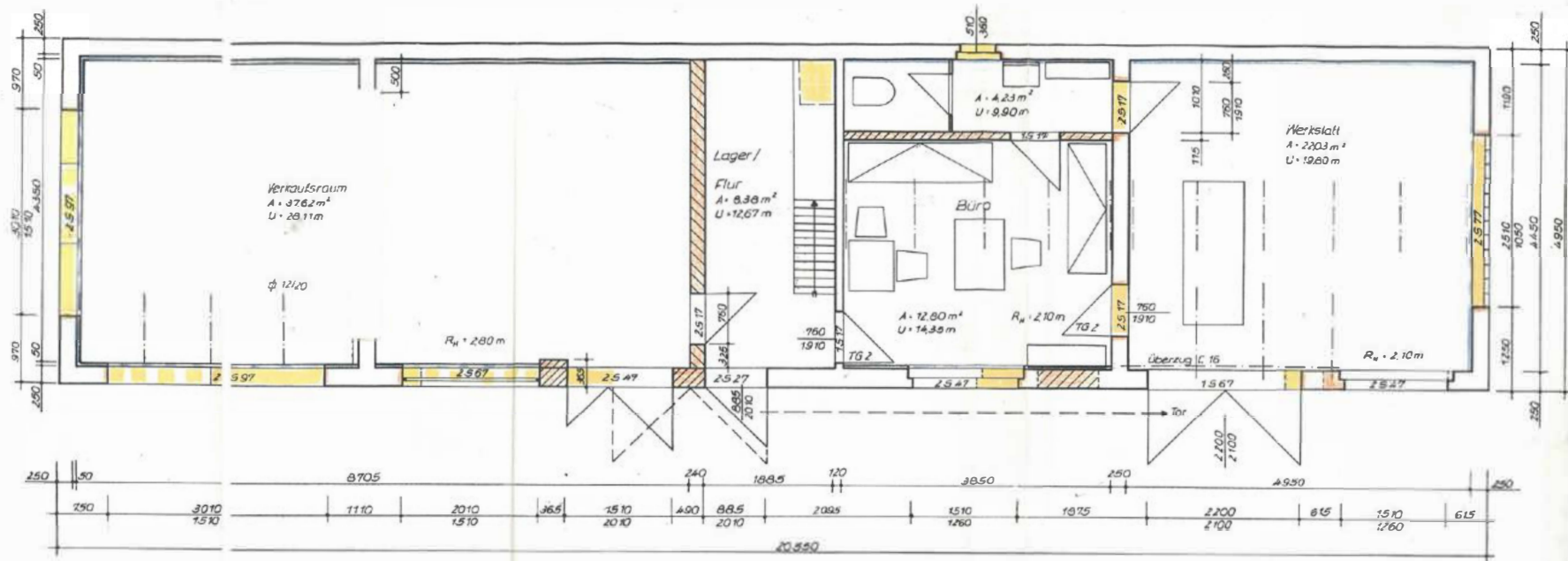
Grundriß
